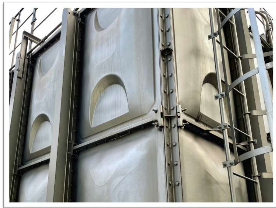
JR田町駅に隣接する新田町ビル、95tの受水槽（設置38年目）
